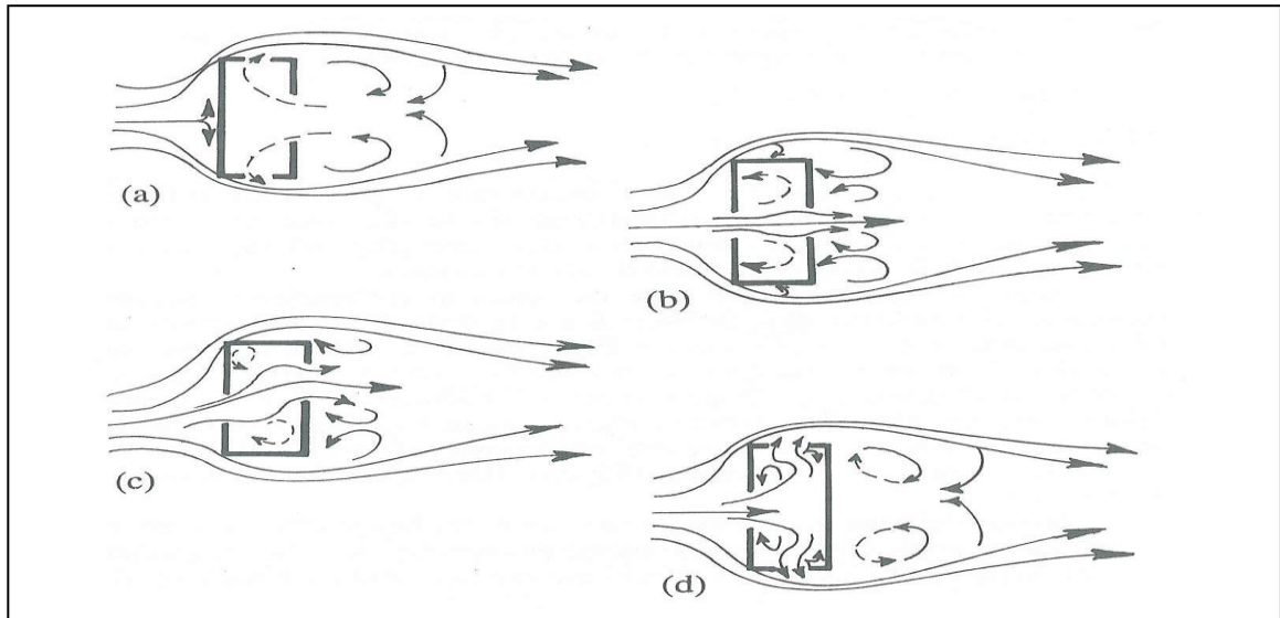
SCHEMA 2 – Posizionamento orizzontale di aperture, in funzione della ventilazione passante – vento obliquo alle facciate dell'edificio
