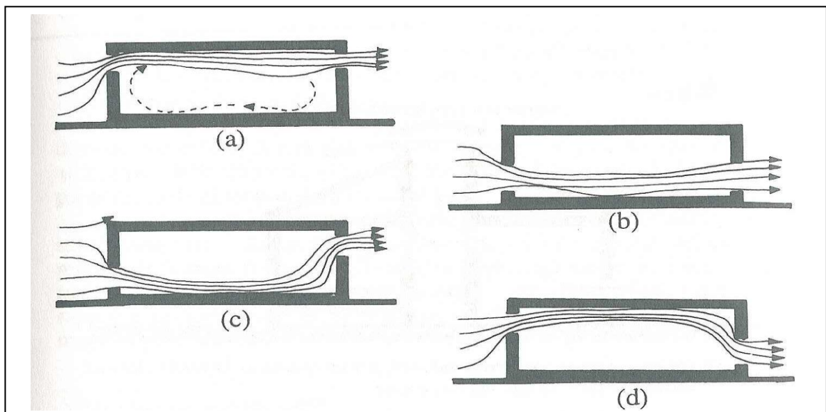
SCHEMA 3 – Flusso d'aria interno ad un ambiente, in funzione della collocazione verticale delle aperture, nel caso di ventilazione passante
