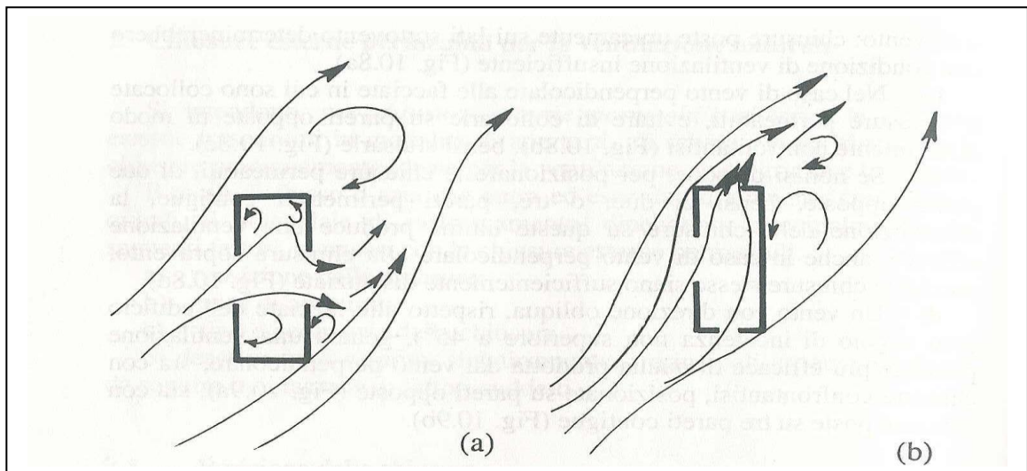
SCHEMA 3 – Flusso d'aria interno ad un ambiente, in funzione della collocazione verticale delle aperture, nel caso di ventilazione passante
